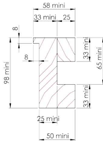
Profil une aile de recouvrement
