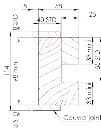
Profil avec 2 couvre-joints
