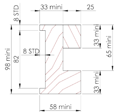
Profil rainure à cloison
