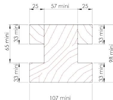
Traverse intermédiaire / Meneau
